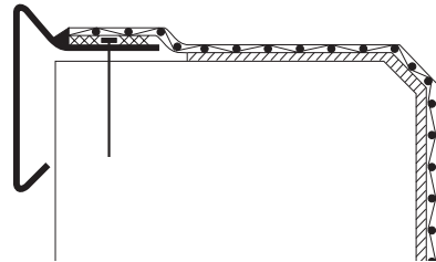
Fig. 4: Encolado en su totalidad
