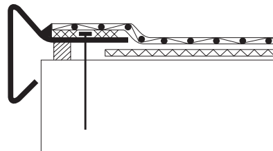
Fig. 5: Utilización de una junta de compresión RENOLIT ALKORPLUS 81058
